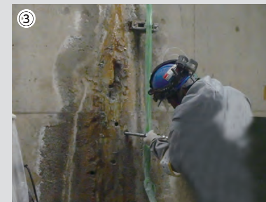
③ 注入ノズルのセット
