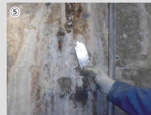
⑤ 急結セメント充填
