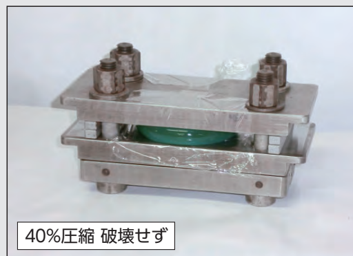
● バンデフレキシソソ圧縮試験
